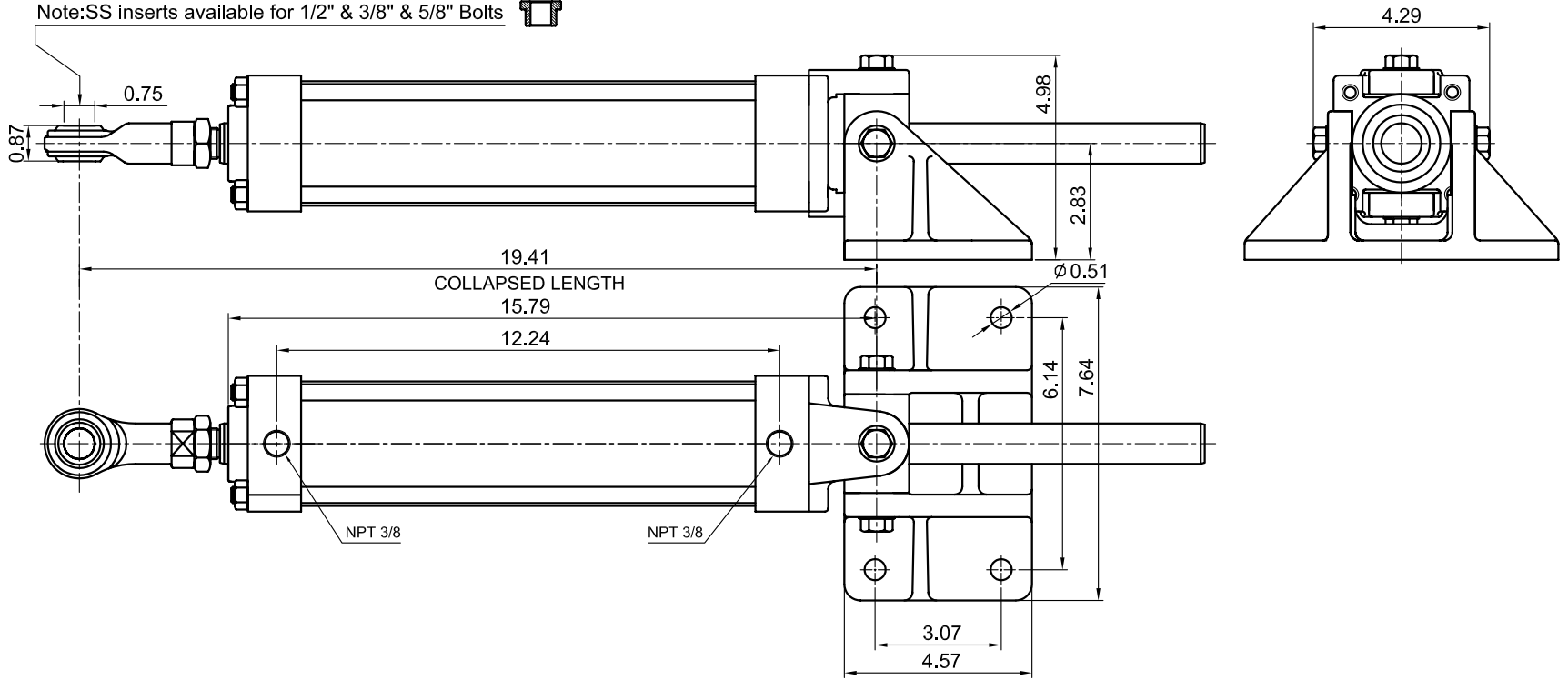
Model : HC250B-9 35°
