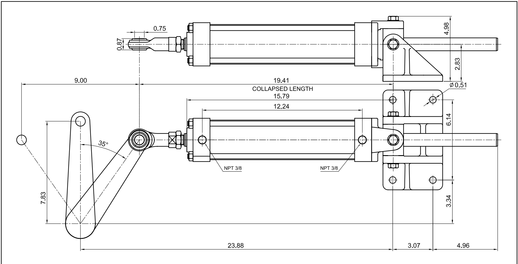
Model : HC250B-9 35°
