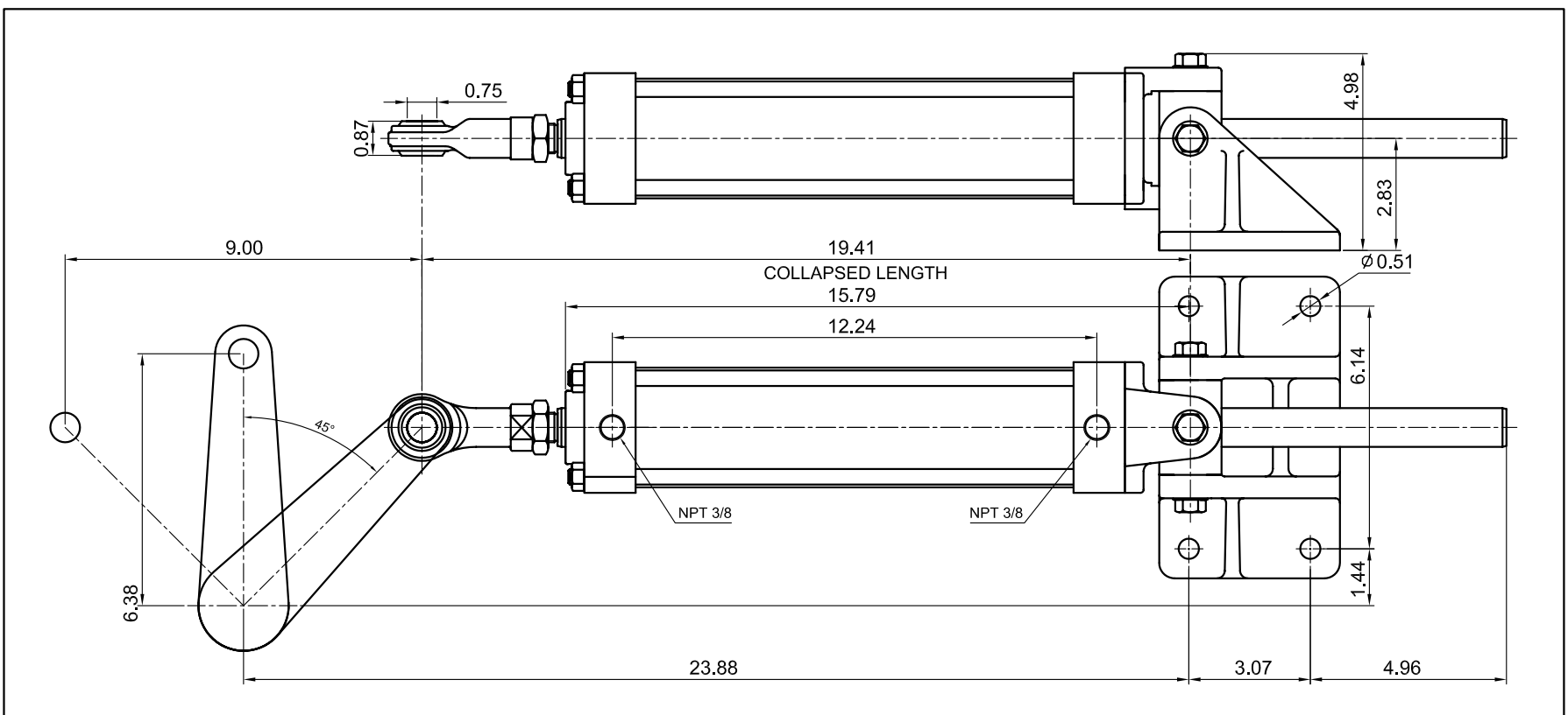
Model : HC250B-9 45°
